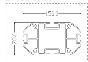
L Alu.Profile
